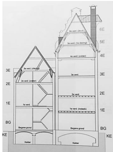
Afb. 5. Dwarsdoorsnede van het huis dat laat zien hoe groot dit huis is (uit het waardestellend rapport p. 12).
